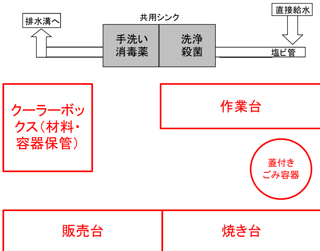
開設予定施設平面図
